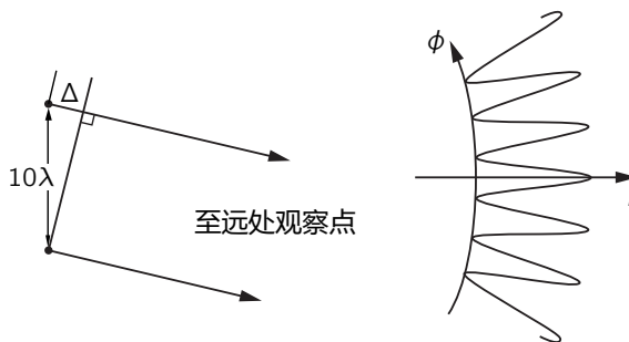
图 29.7: 两个相聚 10\lambda 的偶极子的强度分布图
