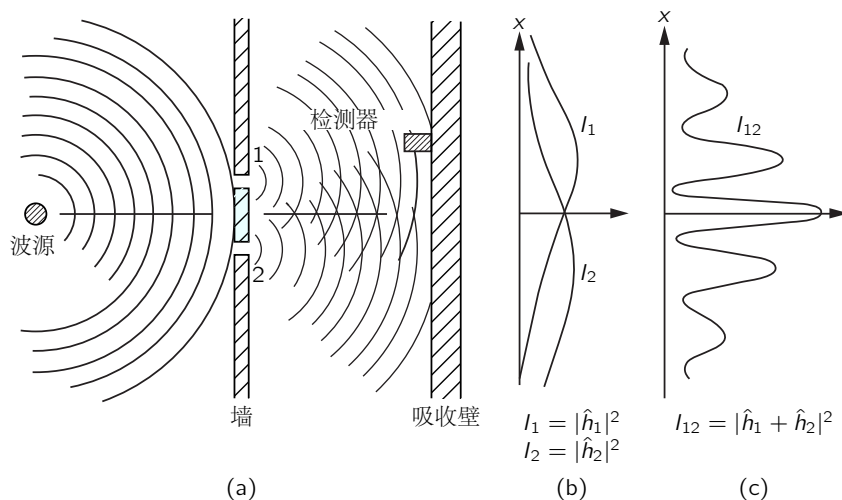
图 37.2: 水波的干涉实验
