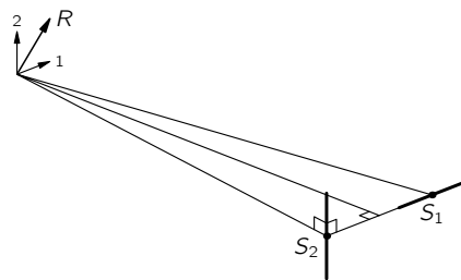
图 28.4: 两个源叠加时的矢量特征示意图
