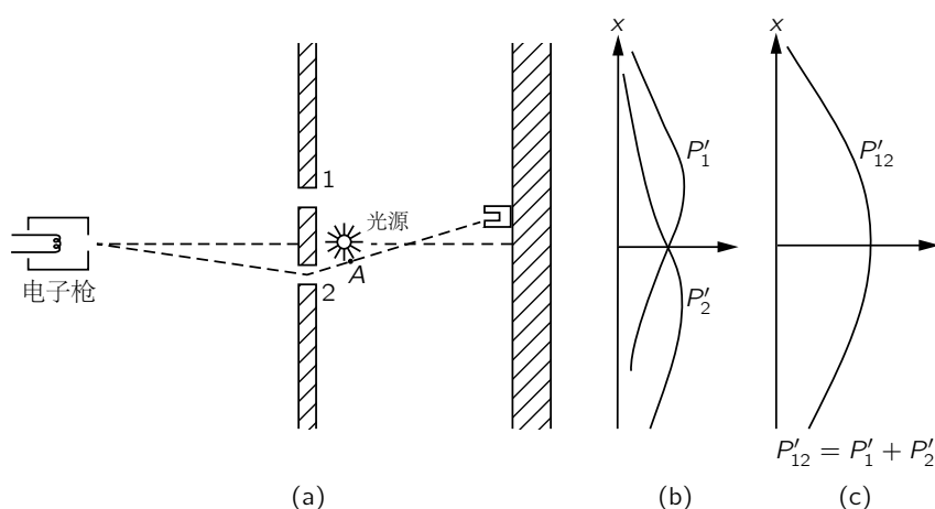
图 37.4: 另一个电子的实验
