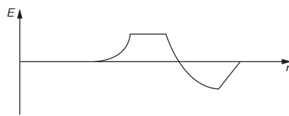
图 29.3: 下一时刻的电场与位置的关系 (忽略 1/r 引起的改变)
