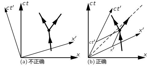
图 17.2: 对一个蜕变粒子的两种看法
