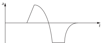
图 29.2: 某电荷的加速度与时间的关系
